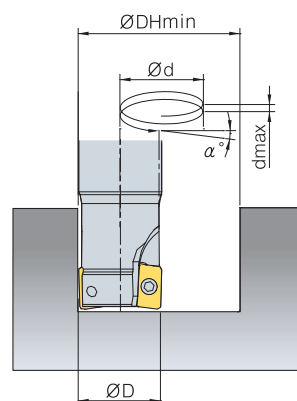
3. Винтовое врезание для сквозных отверстий
