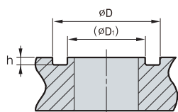
Фрезерование канавки под уплотнительное кольцо
