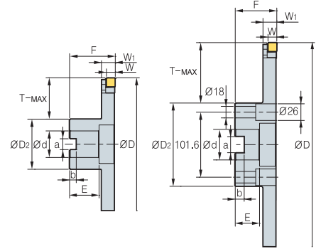
ØD : Ø100~Ø200
