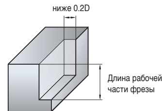
3. Фрезерование уступов
